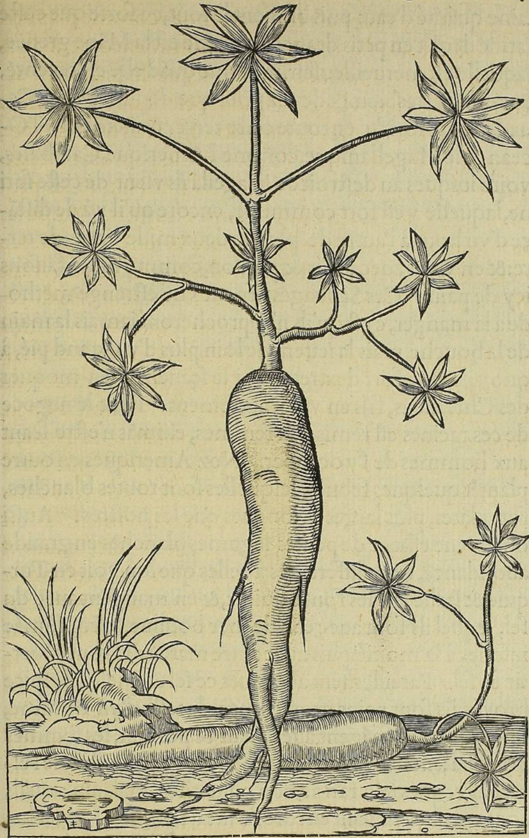
F ij
