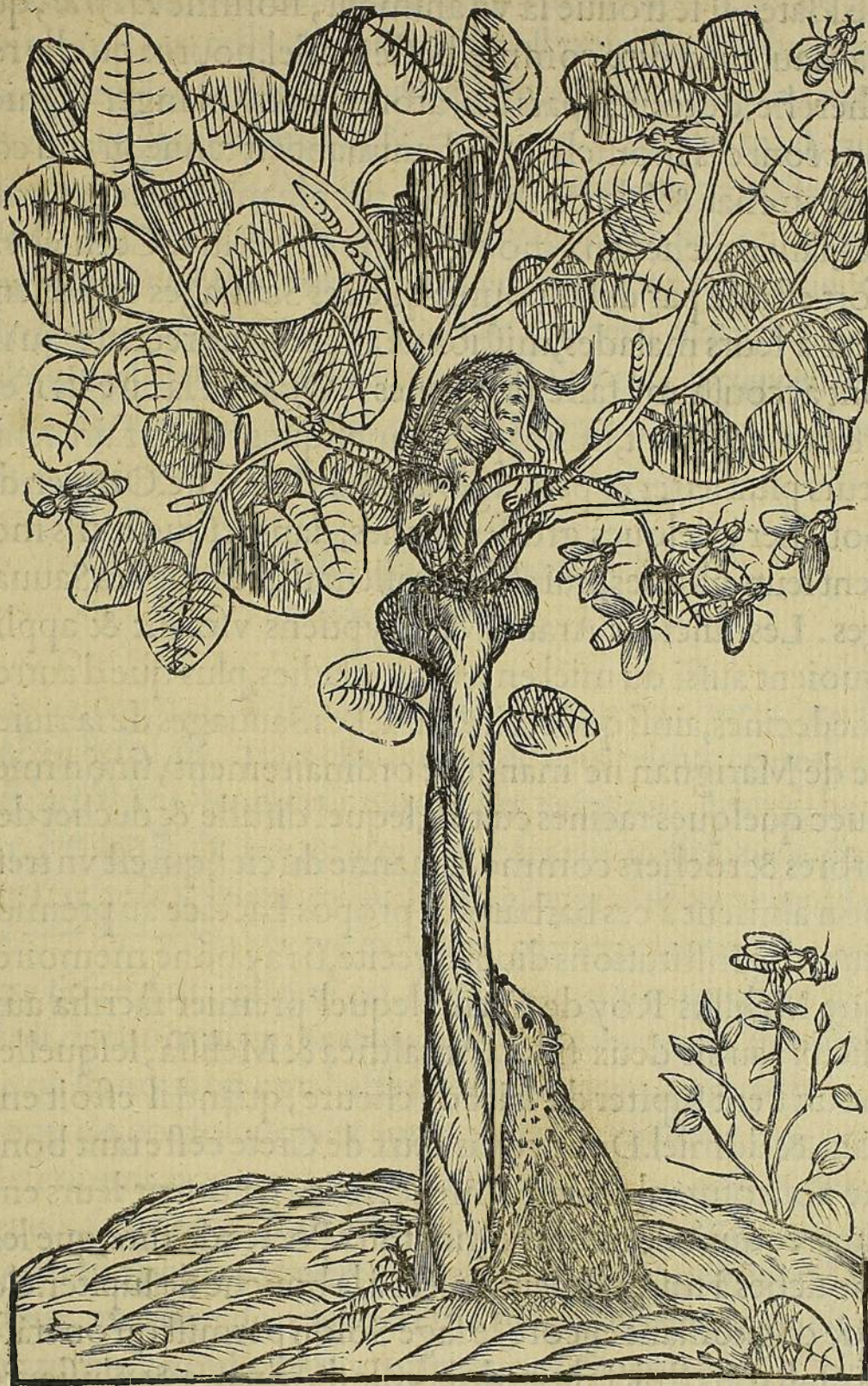
B ij
